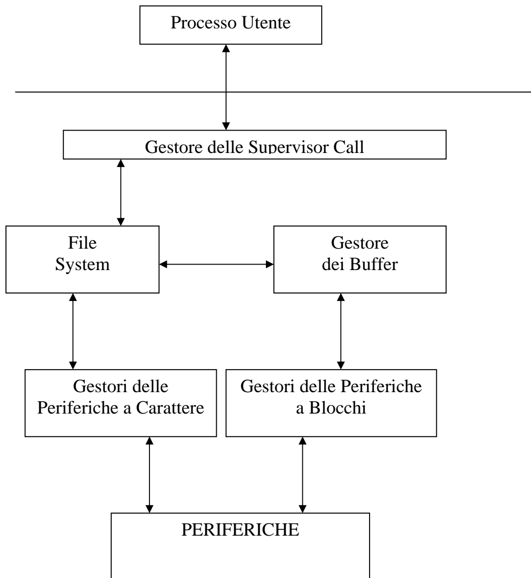
Figura 1 – Gestori delle periferiche a blocchi e a carattere
